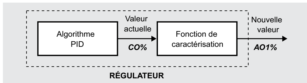
Figure 4.5 Régulateur avec fonction de caractérisation
